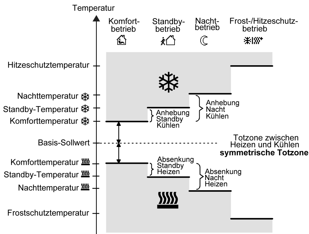
Bild 41: Solltemperaturen in der Betriebsart "Heizen und Kühlen" mit symmetrischer Totzone
