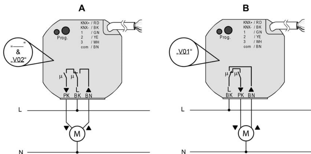
Bild 4: Anschluss der Netzspannung und der Last (abhängig von der Versionskennzeichnung)
