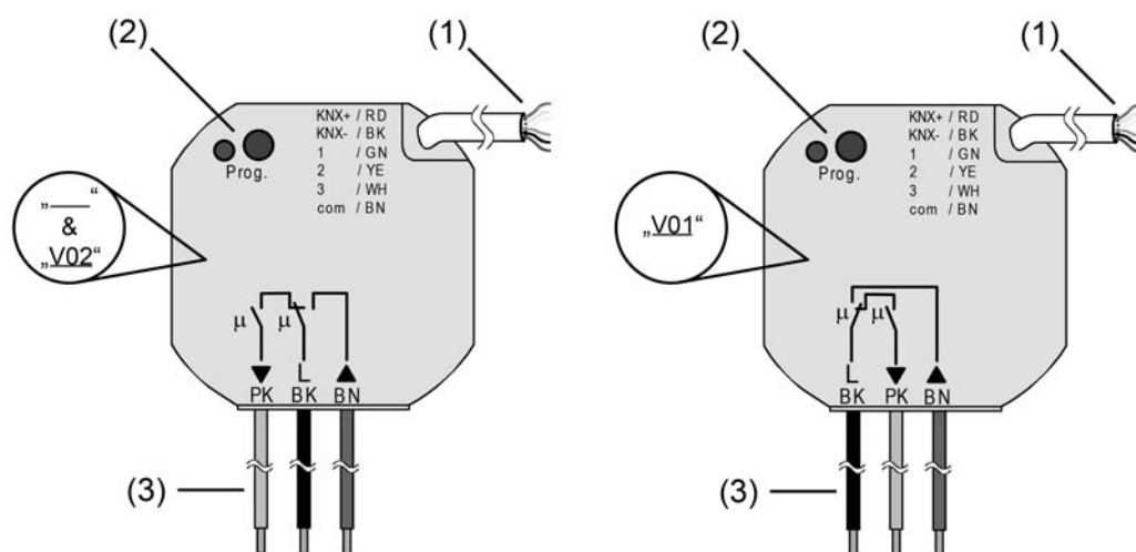
Bild 1: Geräteaufbau
